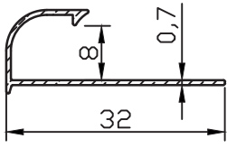
FC-9888 0.103 kg/m
