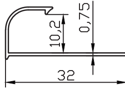
FC-9887 0.113 kg/m
