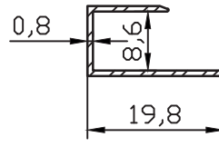
PR-9555 0.086 kg/m
