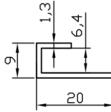
PR-9012 0.124 kg/m
