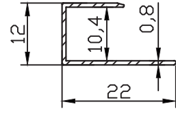
PR-10181 0.095 kg/m
