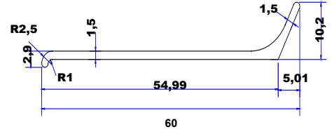
SP-2002 0,279kg/m
