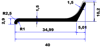
SP-2001 0,198kg/m
