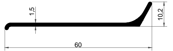
KF-1072 0.279 kg/m
