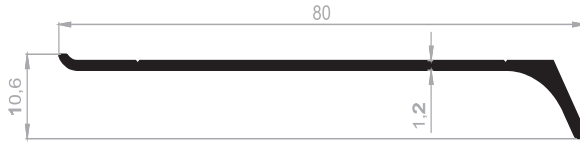
SP-2003 0,310 kg/m
