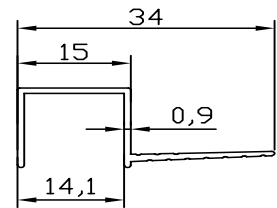
FC-10012 0.144 kg/m
