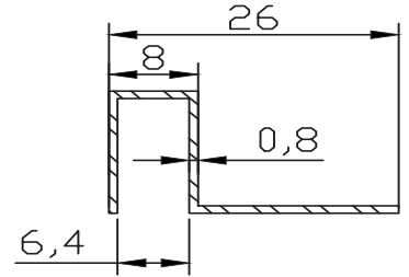
FC-5233 0.111 kg/m
