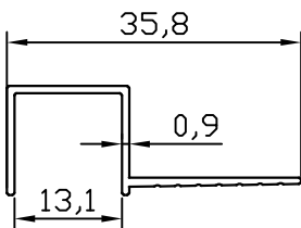
FC-10165 0.146 kg/m
