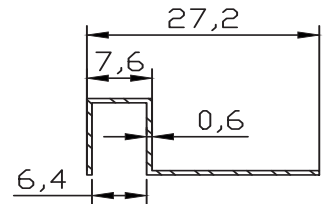
FC-5221 0.076 kg/m
