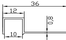
FC-5324 0.141 kg/m
