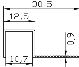
FC-10172 0.133 kg/m
