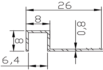
FC-5231 0.092 kg/m
