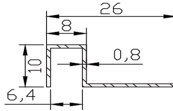
FC-5232 0.100 kg/m
