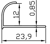
FC - 10285 0.095 kg/m
