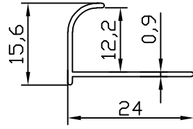
FC - 5342 0.103 kg/m
