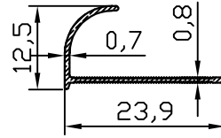
FC - 10503 0.073 kg/m
