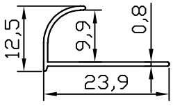
FC - 10087 0.087 kg/m
