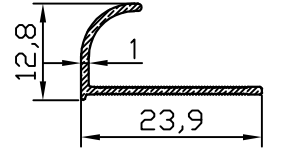
FC - 10509 0.100 kg/m
