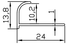
FC - 5341 0.108 kg/m
