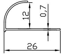
FC - 10014 0.087 kg/m
